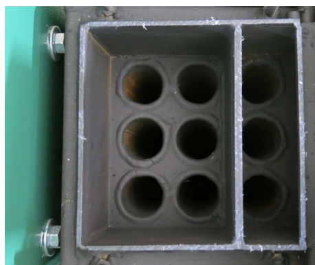
Рис. 8 - Доступ к прочистной крышке теплообменника
